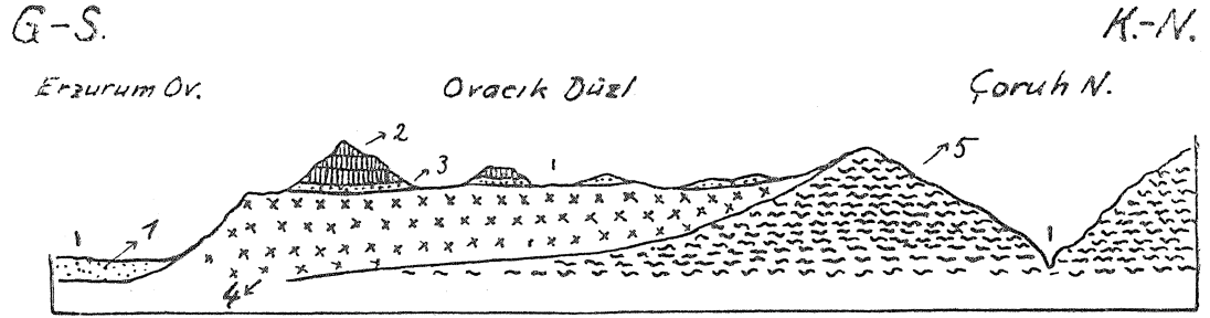
Şekil 1. — Fig. 1. Ovacik düzlüğünün şematik makta! (Erzurum ovası ile Çoruh vâdisi arasında) — Coupe schématique du plateau cOvacik (entre la plaine d'Erzurum et la vallée du Çoruh Nehri).
