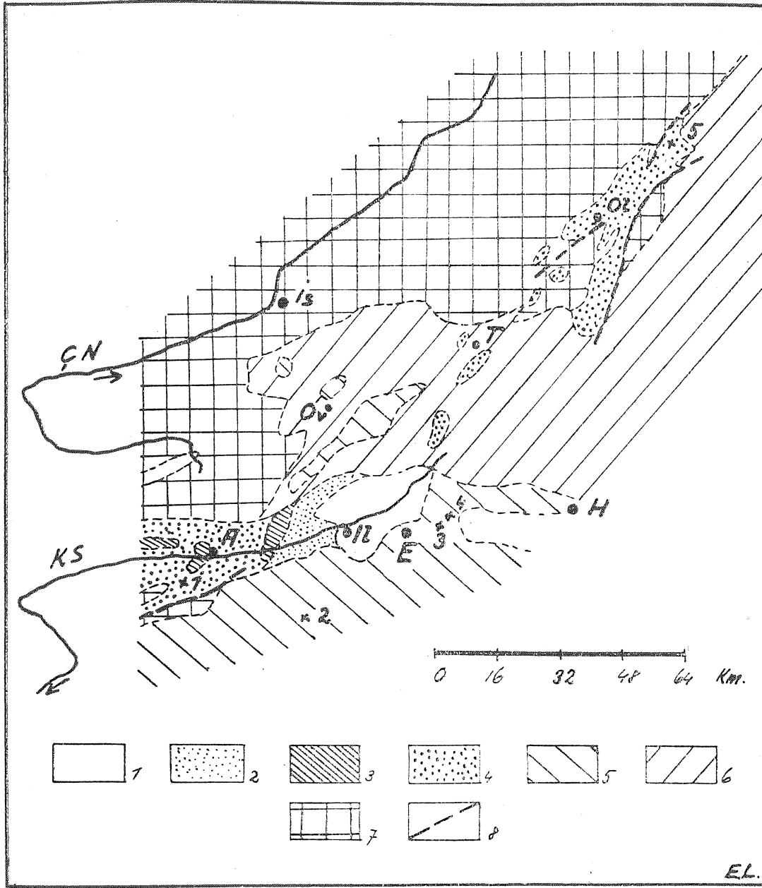
Şekil 4. — Fig. 4. Erzurum-Oltu-Ispir havalisinin jeolojik krokisi — Croquis géologique de la région d'Erzurum-Oltu-Ispir.
