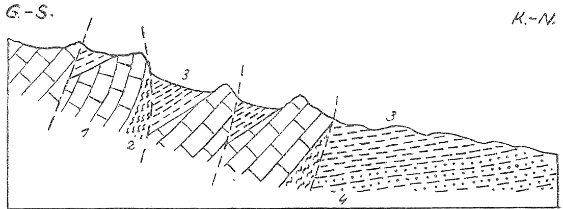
Şekil 2. — Fig. 2. Kükürtlü havzasındaki Oligosen tabakalarının parçalanmasını gösteren bir makta — Coupe montrant le morcellement des terrains oligocènes dans le bassin de Kükürtlü.
