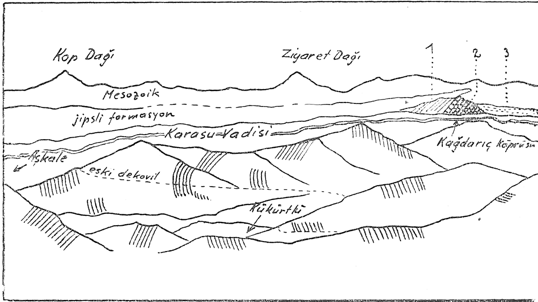
Şekil 3. — Fig. 3... Akbaba Dağından Karasu vâdisine doğru bakış; Öliosen arazisinin gayri muntazam iltivalanması ve Kağdarıç'taki anormal kontakt. — Vue le FAkbaba Dağı vers la vallée du Karasu; plissement irrégulier des terrains oligocènes et le contact anormal de Kağdarıç.
